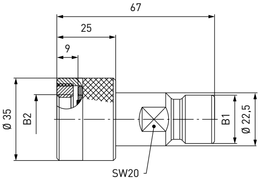
TW04 CNG mit integriertem Absperrventil
