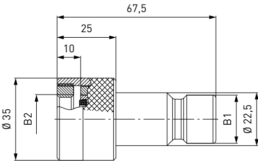
TW04 CNG ohne integriertes Absperrventil
